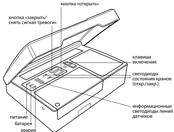
Рис. 2. Вид модуля управления Neptune ProW с открытой крышкой.
